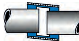
Rohrversatz von bis zu 10 mm
