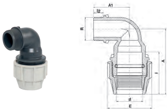
Abbildung und technische Zeichnung für die Dimensionen 20 mm bis 63 mm
