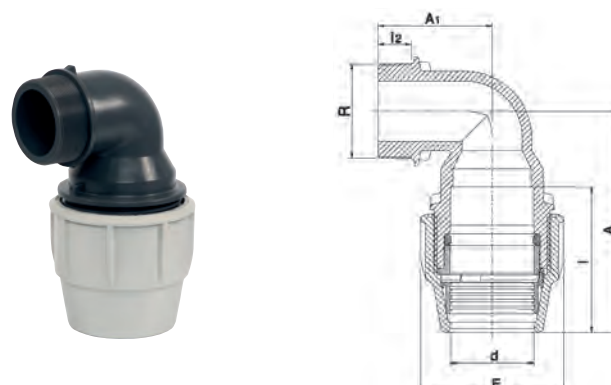
Abbildung und technische Zeichnung für die Dimensionen 75 mm bis 110 mm
