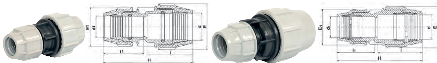
Abbildung und technische Zeichnung für die Dimensionen 16 mm bis 63 mm
